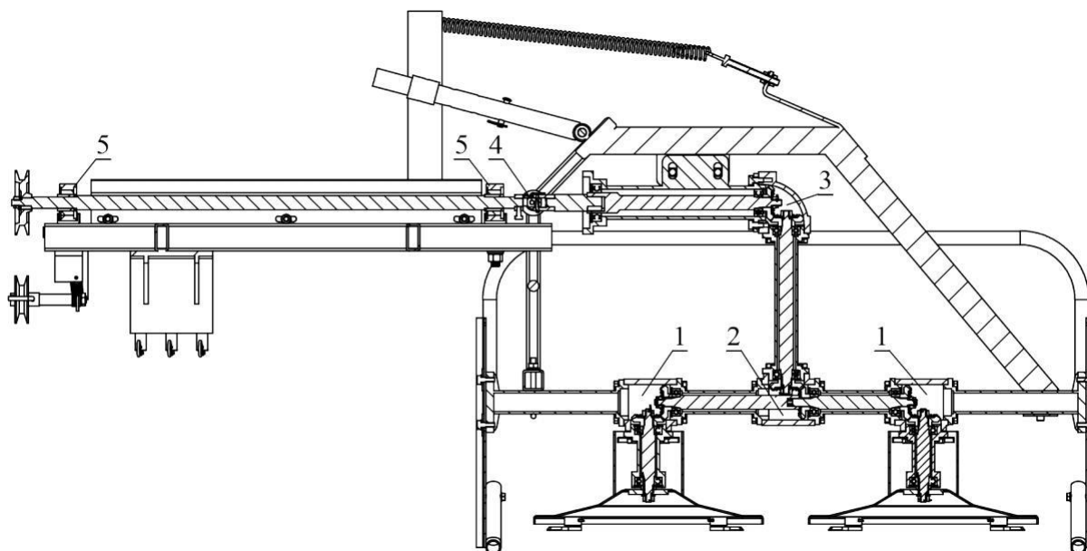
Рис. 2. Места смазки задней роторной косилки KP3-T2
