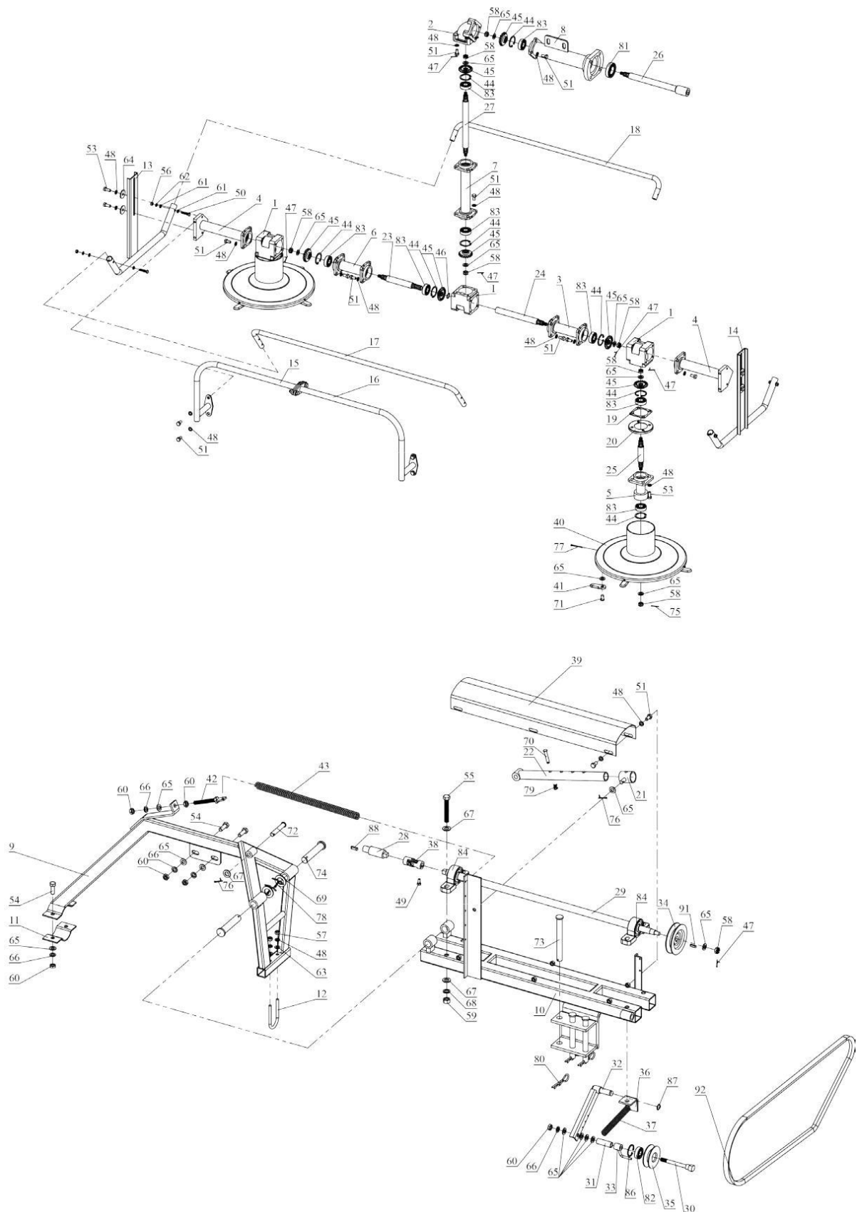
Рис. 3. Комплектующие задней роторной косилки КРЗ-Т2 к мини-тракторам КЕНТАВР
